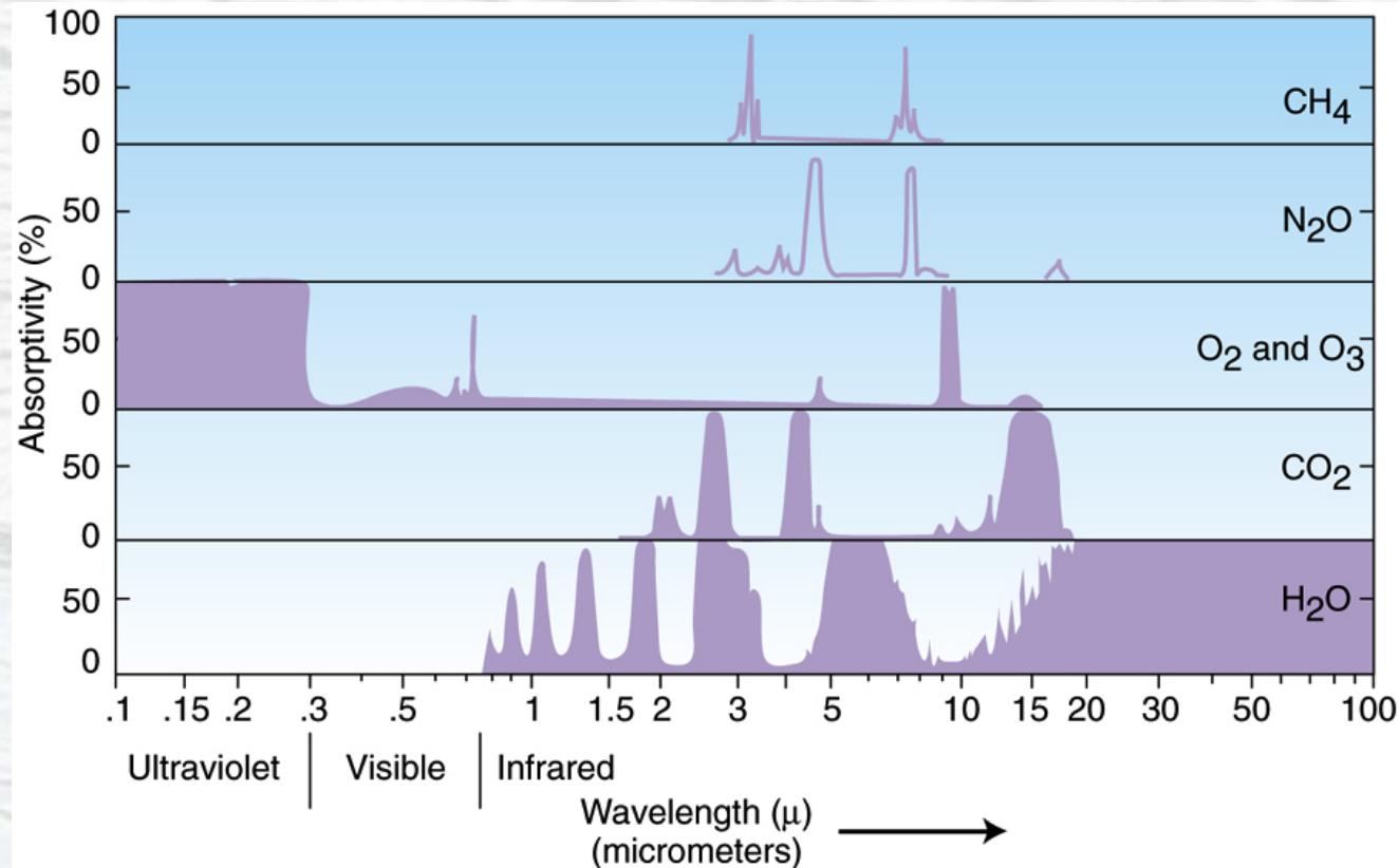
Figura. Absorción de energía por distintos gases como función de la longitud de onda.
