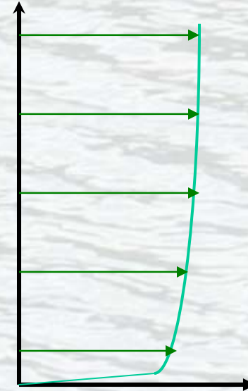
Perfil de rapidez del viento para una superficie sin rugosidad pero con una débil fricción
